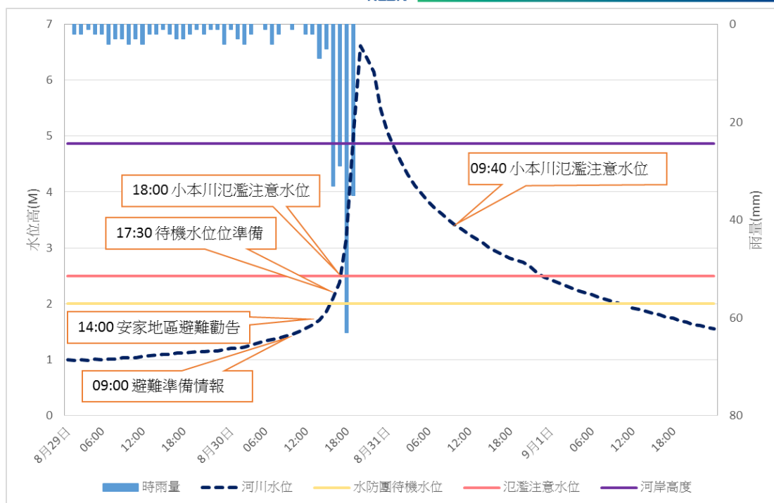
圖 4-小本川赤鹿橋水位歷線與延泉町雨量組體圖
